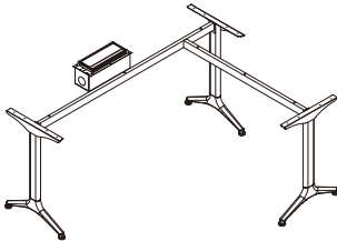
R-60-J1608A 1600*800*760 R-60-J1809A 1800*900*760
