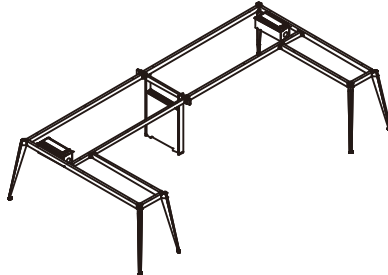
R-73-2L2412 2400*1200*760 R-73-2L2814 2800*1400*760
