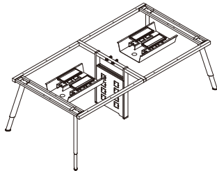
R-80-2412-4 2400*1200*800 R-80-2814-4 2800*1400*800
