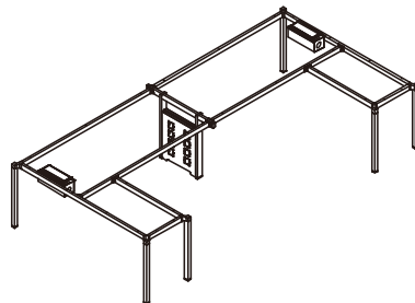
R-82-2L2412 2400*1200*800 R-82-2L2814 2800*1400*800
