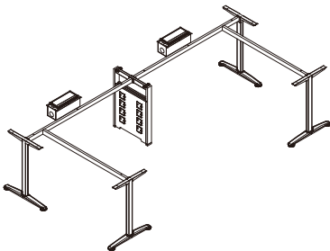
R-98-2L2412 2400*1200*760 R-98-2L2814 2800*1400*760
