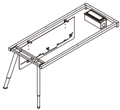
R-80-J1608B 1600*800*800 R-80-J1809B 1800*900*800
