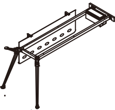
R-77-J1608B 1600*800*770 R-77-J1809B 1800*900*770
