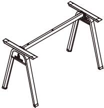
R-08-J1608C 1600*800*750 R-08-J1809C 1800*900*750
