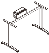
R-98-J1608B 1600*800*760 R-98-J1809B 1800*900*760
