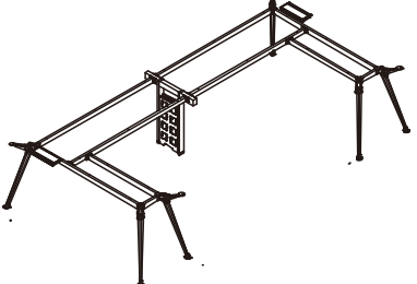
R-77-2L2412 2400*1200*770 R-77-2L2814 2800*1400*770
