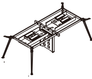
R-77-2412-4 2400*1200*770 R-77-2814-4 2800*1400*770
