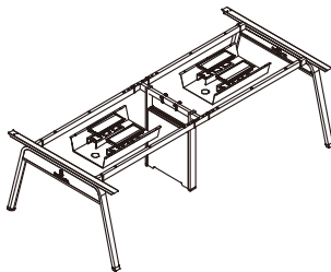
R-08-2412-4 2400*1200*750 R-08-2814-4 2800*1400*750
