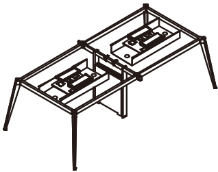
R-73-2412-4 2400*1200*760 R-73-2814-4 2800*1400*760
